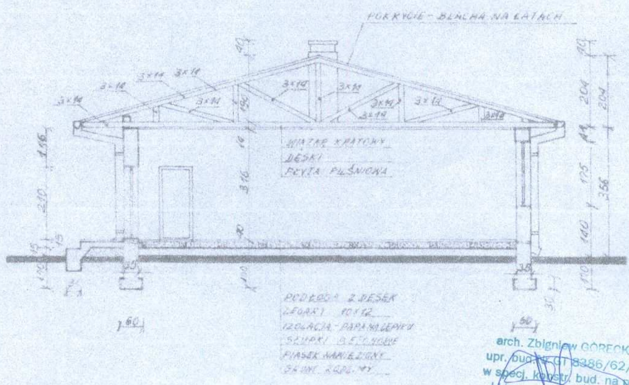
PRZEKROJ B-B 1:100
