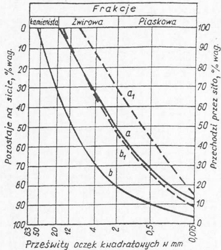
Rysunek 1. Obszar uziarnienia optymalnych mieszanek żwirowych
