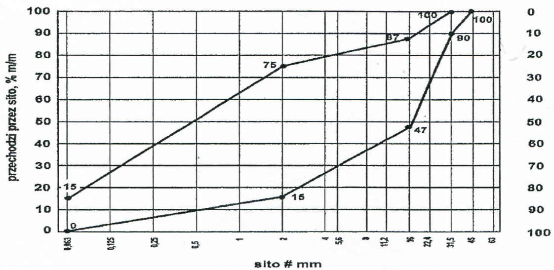
Rys. 19. Mieszanka niezwiązana 0/31,5 do nawierzchni z kruszywa niezwiązanego
