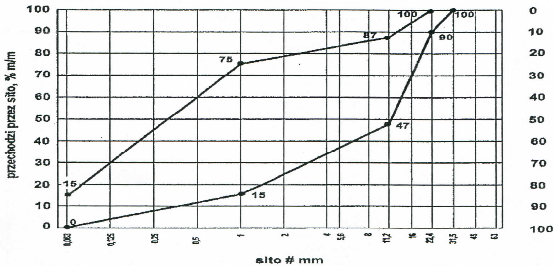
Rys. 18. Mieszanka niezwiązana 0/22,4 do nawierzchni z kruszywa niezwiązanego
